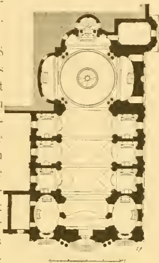
Fig. 59. St. Nikolauskirche zu Prag (Kleinſeite). Grundriß.
